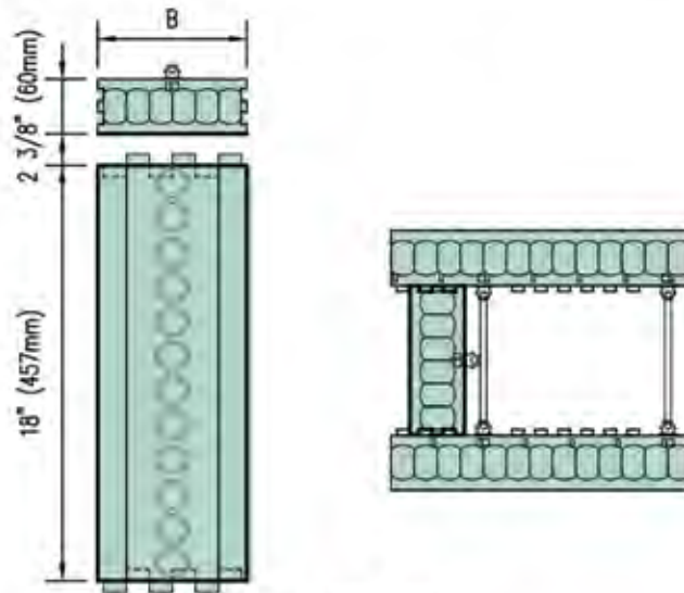
END CAP
